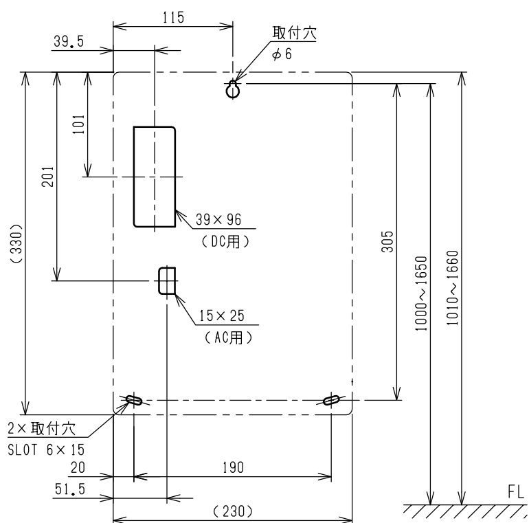
通線穴位置および取付穴位置 (正面図)
